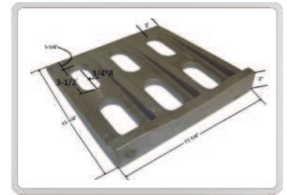
DA Pt # DA-81777 Alt Pt # 578106-0 Description: Draft Lug - Front
